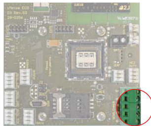
iMETOS ECO D3
